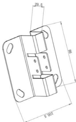
Wymiary płyty montażowej
