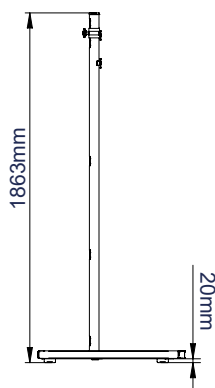
WIDOK Z BOKU WOLNOSTOJĄCY
