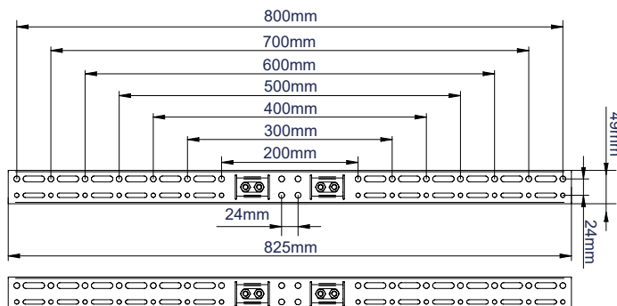
MOCOWANIE DLA ROZMIARU DO 800MM
