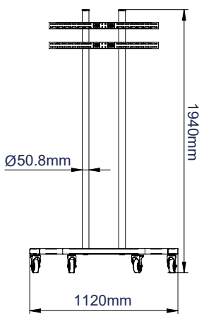
WIDOK Z PRZODU Z KÓŁKAMI
