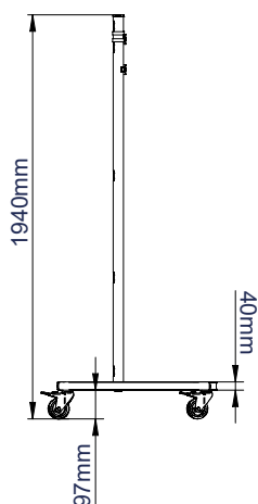
WIDOK Z BOKU Z KÓŁKAMI
